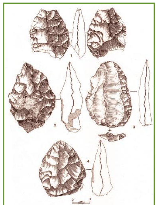
Bifaces (1-2 et 4) et racloir (3) trouvés sur le site de Toulousète à Beauville
